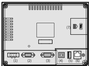
后视图
